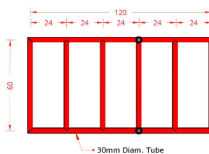
LADDER - PLAN scale: 1:25
