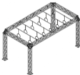
RINGS - ISO STRUCTURE SCALE: 1:100
