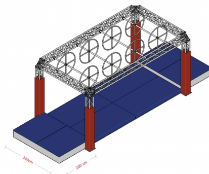
WHEELS - ISO COMPLETE scale: 1:25
