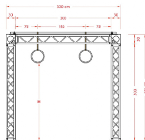
RINGS - ISO STRUCTURE SCALE: 1:100
