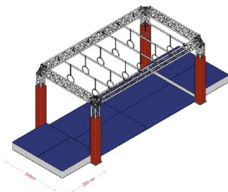
RINGS - ISO COMPLETE SCALE: 1:100
