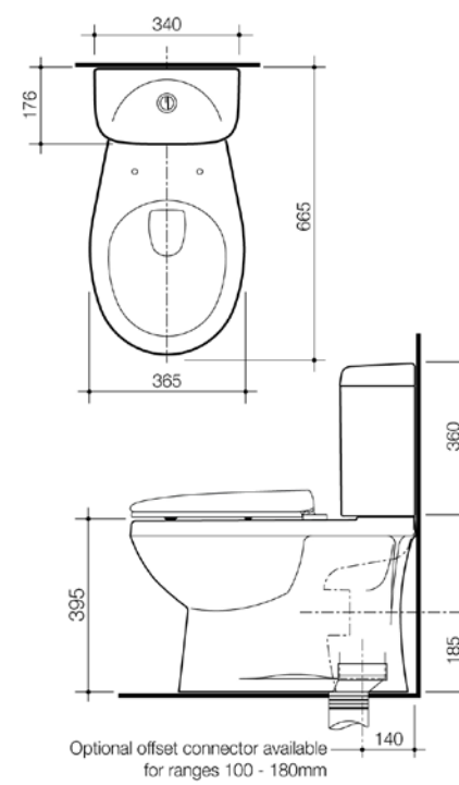
VENECIA CC 4S SNV SUITE SC
