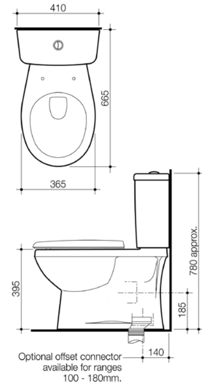
STYLUS BASIS BTW CC 4S BI SUITE
