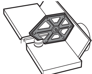
Figure 3 : Utilisation avec un guide de dégauchisseuse
