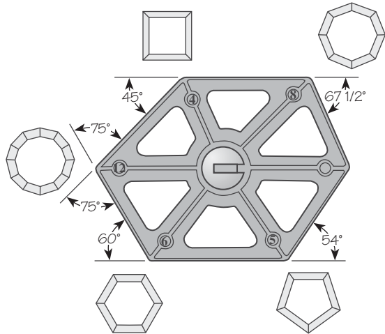
Figure 1 : Angles courants du gabarit polyvalent
