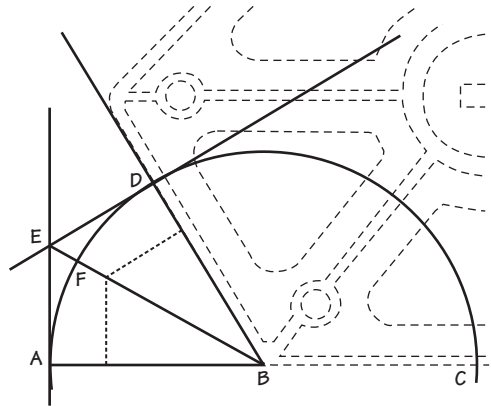
Figure 6 : Utilisation du gabarit pour le traçage
