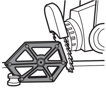
Figure 5 : Réglage de l'inclinaison de la lame d'une scie radiale
