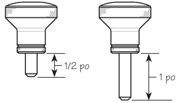
Figure 1 : Configuration de la molette de blocage
