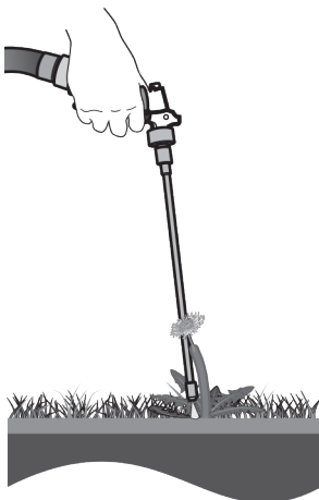
Figure 2 : Insertion de la désherbeuse hydraulique
