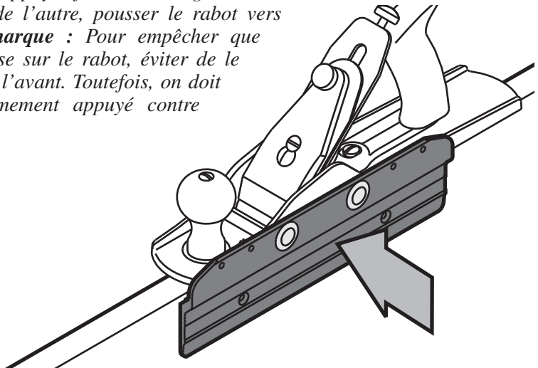
Figure 3 : Le guide est plaqué fermement contre la pièce.
