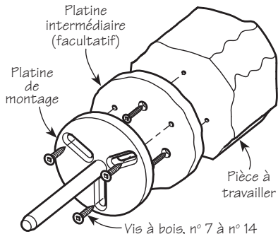
Figure 6 : Fixer une sculpture sur la platine de montage en utilisant une pièce de bois intermédiaire
