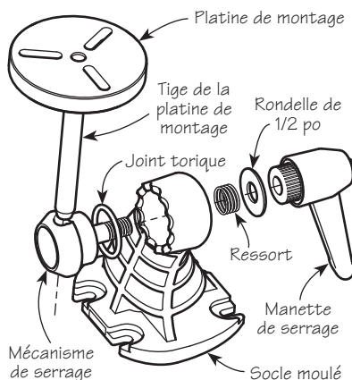
Figure 7 : Vue éclatée de l'étau de sculpteur
