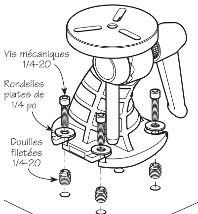
Figure 3 : Étau de sculpteur fixé à l'aide de douilles filetées
