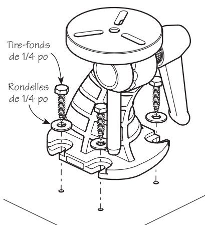
Figure 2 : Étau de sculpteur fixé à l'aide de tire-fonds de 1/4 po
