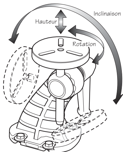
Figure 1 : Platine ajustable sur trois axes
