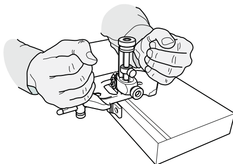
Figure 4 : Utilisation de l'accessoire d'incrustation avec le guide
