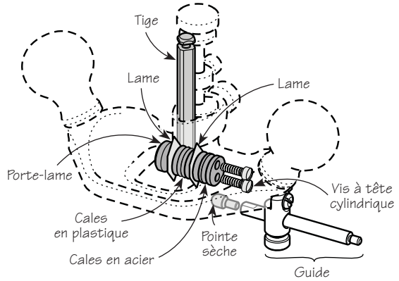
Figure 1 : Composants de l'accessoire d'incrustation – guimbarde non comprise
