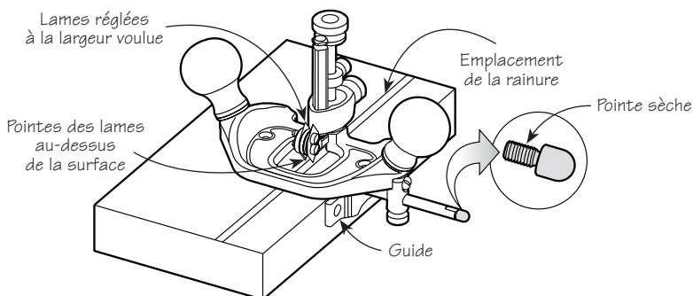
Figure 3 : Configuration pour marquer des rainures droites
