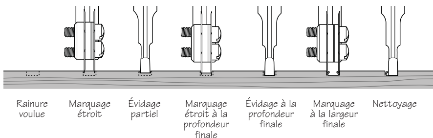
Figure 6 : Réalisation progressive d'une rainure plus profonde
