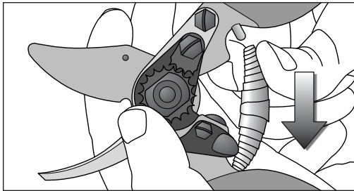
1. Enlevez le ressort.
