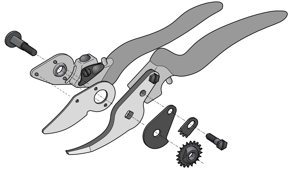
Vue éclatée du sécateur
