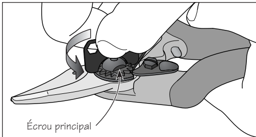
3. Dévisssez puis retirez l'écrou principal et son boulon avec la clé de réglage.
