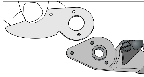
5. Insérez la nouvelle lame et assemblez le tout. Tout en maintenant les poignées fermées, serrez l'écrou principal et la vis de blocage jusqu'à ce qu'il n'y ait plus de jeu entre la lame et l'enclume. Remplacez le ressort entre les poignées. Testez le sécateur pour vous assurer que les pièces n'ont pas été serrées excessivement; ajustez-les au besoin.
