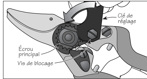
2. À l'aide de la clé de réglage incluse, dévisssez et retirez la vis de blocage.
