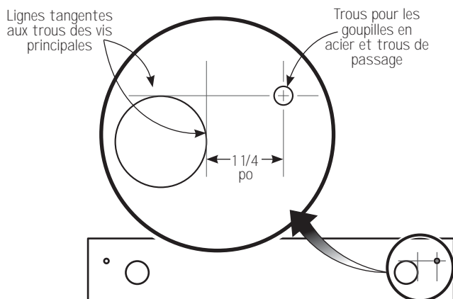
Face intérieure des mâchoires avant et arrière
