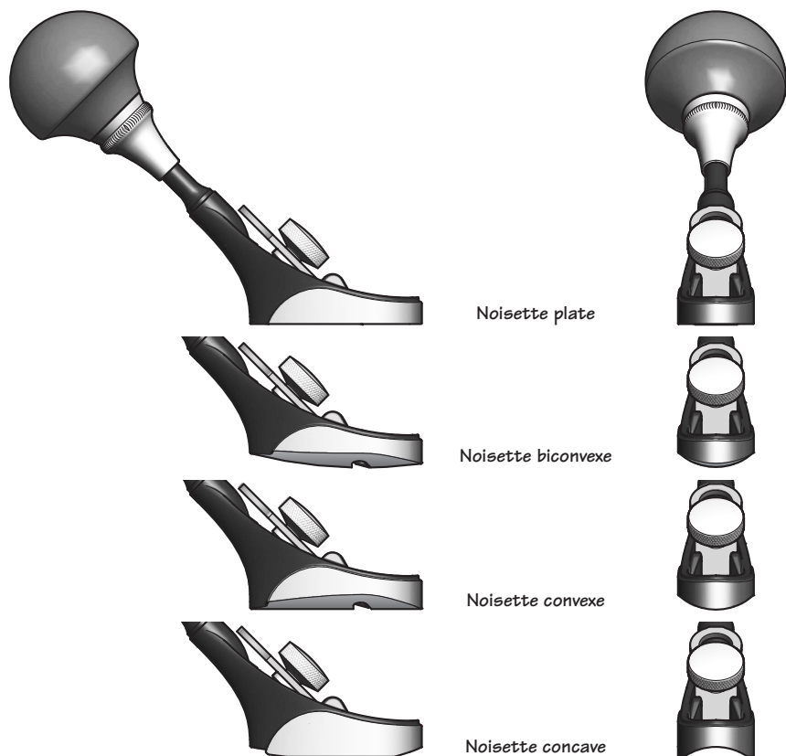
Figure 1 : Les quatre modèles de noisettes à pommeau
