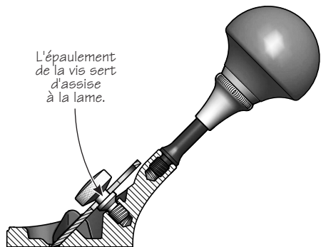
Figure 4 : Blocage de la lame
