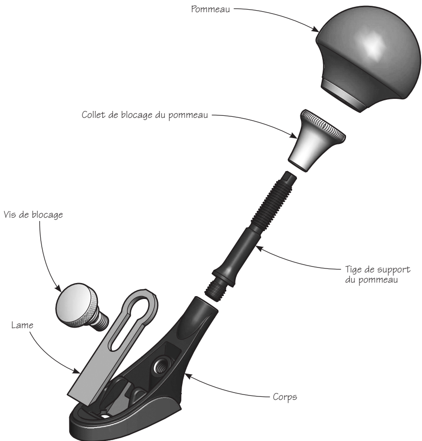
Figure 2 : Vue éclatée d'une noisette
