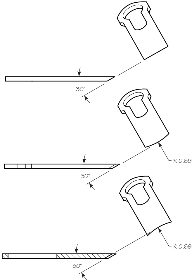
Figure 5 : Affûtage de la lame
