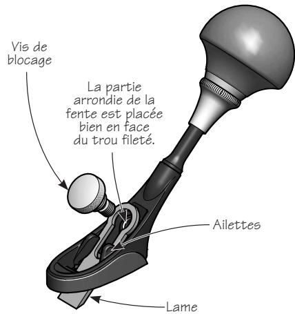
Figure 3 : Montage de la lame
