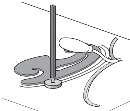
Drawing carving paths. Tracer des motifs à sculpter.
