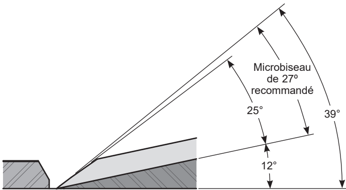
Figure 7 : Géométrie recommandée de la lame du rabot de coupe à angle faible avec un microbiseau de 27^\circ
