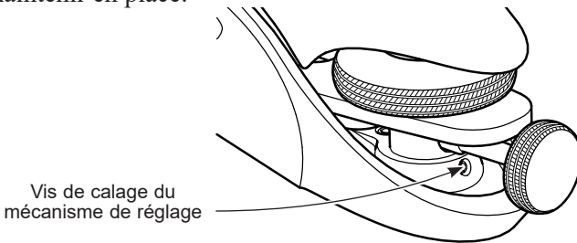
Figure 3 : La vis de calage retient le mécanisme de réglage dans le corps du rabot.
