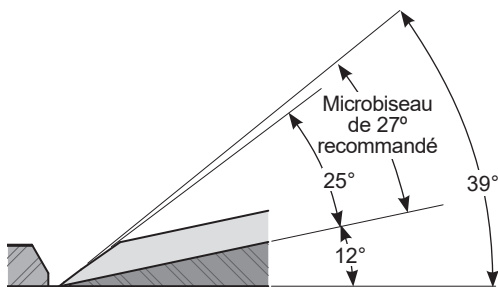
Figure 7 : Géométrie recommandée de la lame du rabot de coupe à angle faible, avec un microbiseau de 27^\circ
