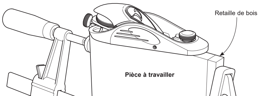
Figure 5 : Prévenir l'éclatement du bois
