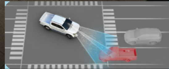
• ระบบเบรกฉุกเฉินอัตโนมัติเมื่อมีรถสวนทางขณะเลี้ยวขวา TA-AEB (Turn Assist with AEB)
