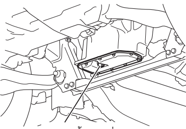
สกรูถ่ายอ่างน้ำมันเครื่อง
